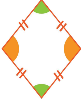
rhombus
